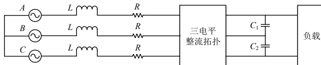
图 2-5 三电平整流器简化结构框图
