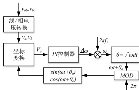
图 2-7 锁相环控制系统框图
