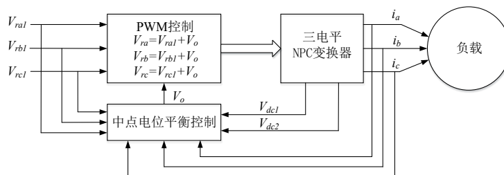
图 3-1 NPC 变换器中点平衡控制框图
